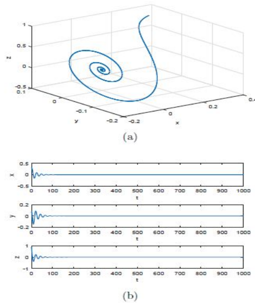
Fig. 3. (a) The phase diagram of the actual system. (b) The actual time diagram of the actual system .
